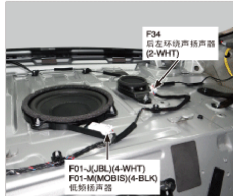
146.后窗台板
